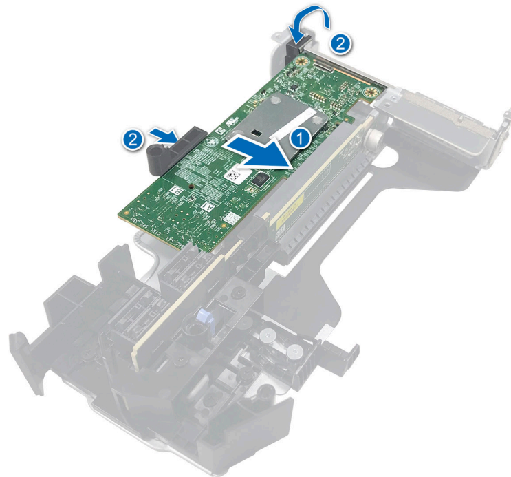
Abbildung 20. Installieren des Dell HBA350i-Adapter
