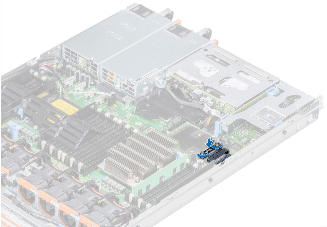
Abbildung 24. Einbauen des Kabels
