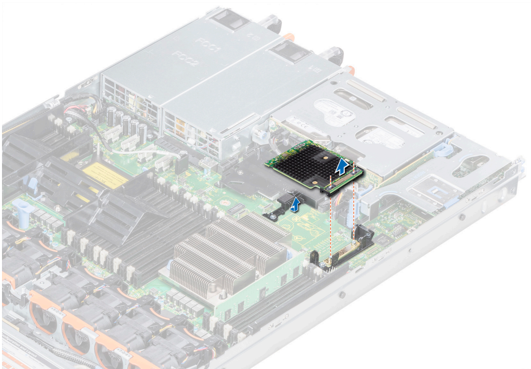
Abbildung 22. Entfernen von HBA350i MM
