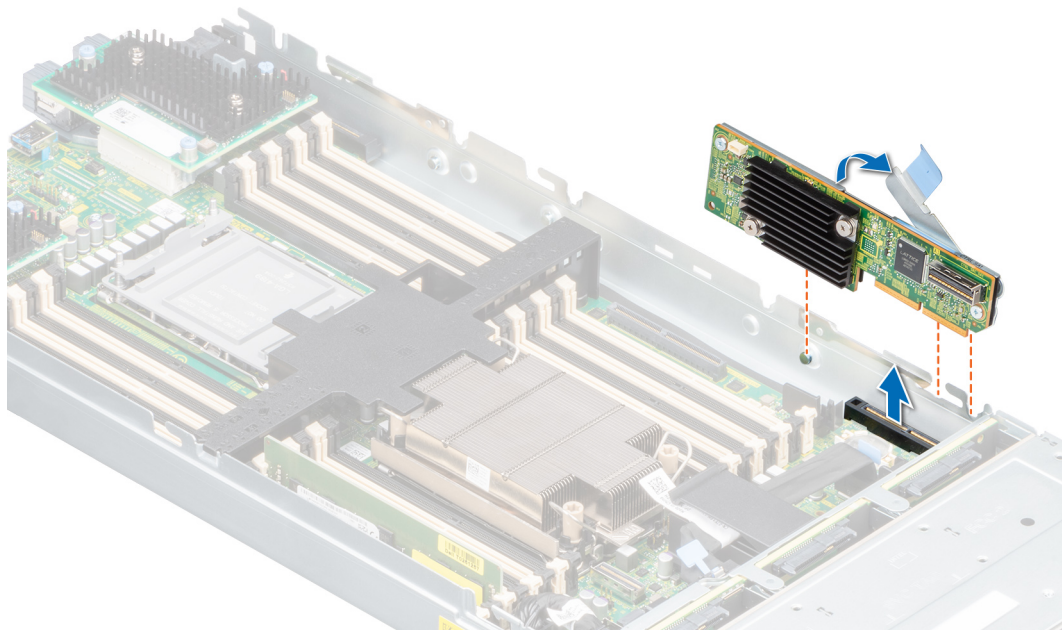
Abbildung 17. Entfernen des Dell HBA350i MX
