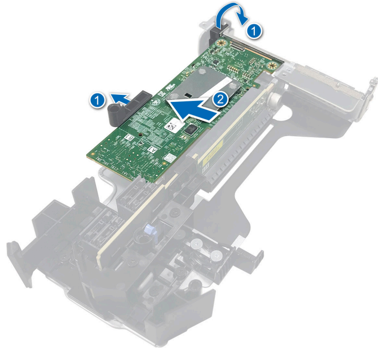
Abbildung 19. Entfernen des HBA350i-Adapter
