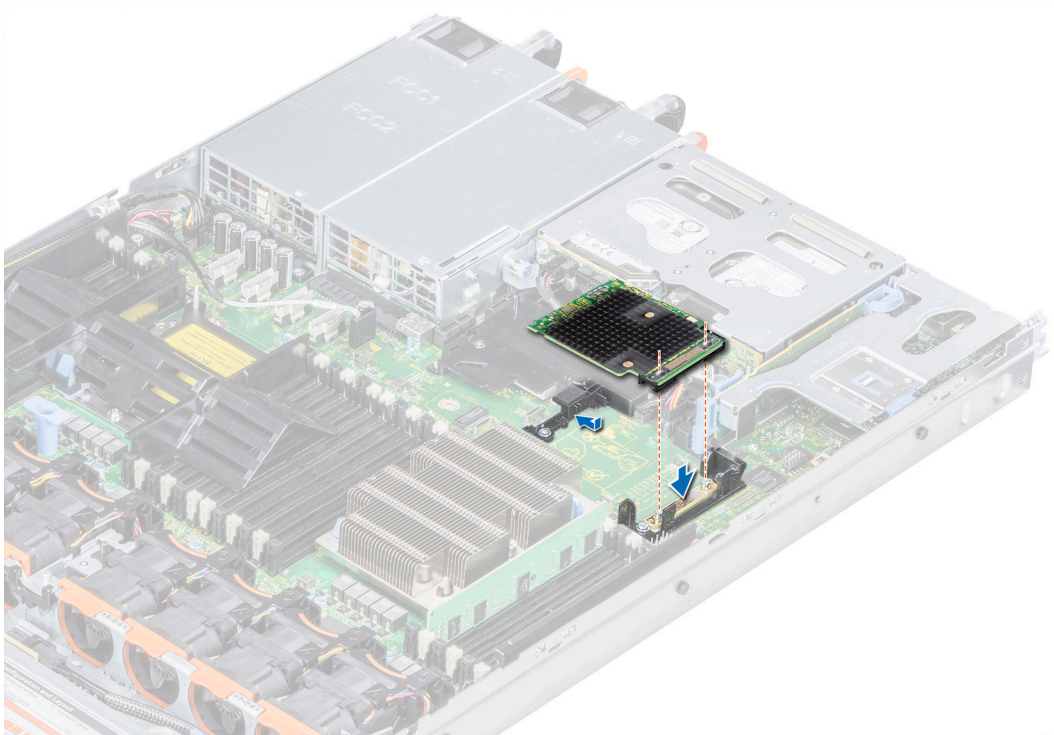
Abbildung 23. Installieren des Dell HBA350i MM
