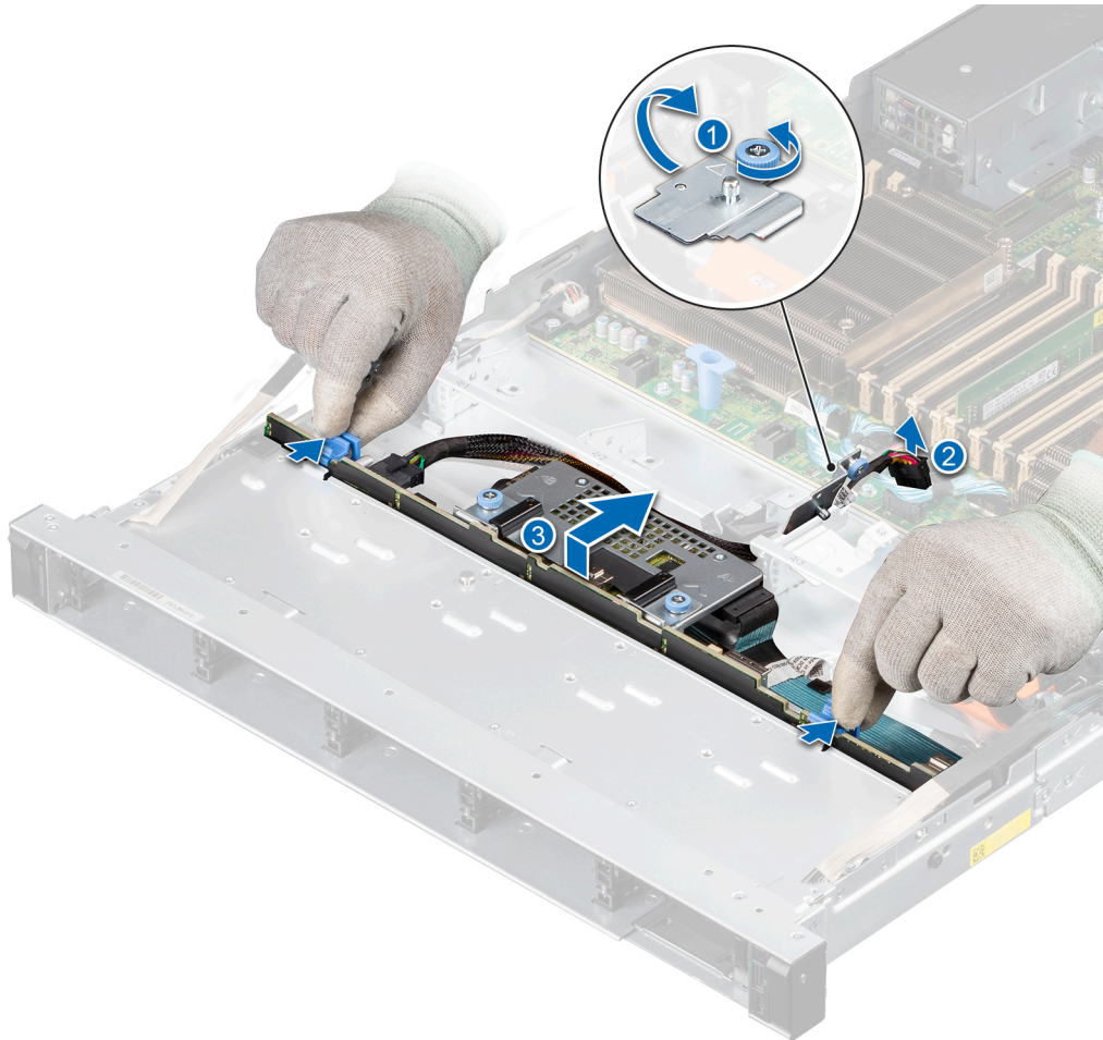
Abbildung 42. Laufwerkrückwandplatine entfernen
