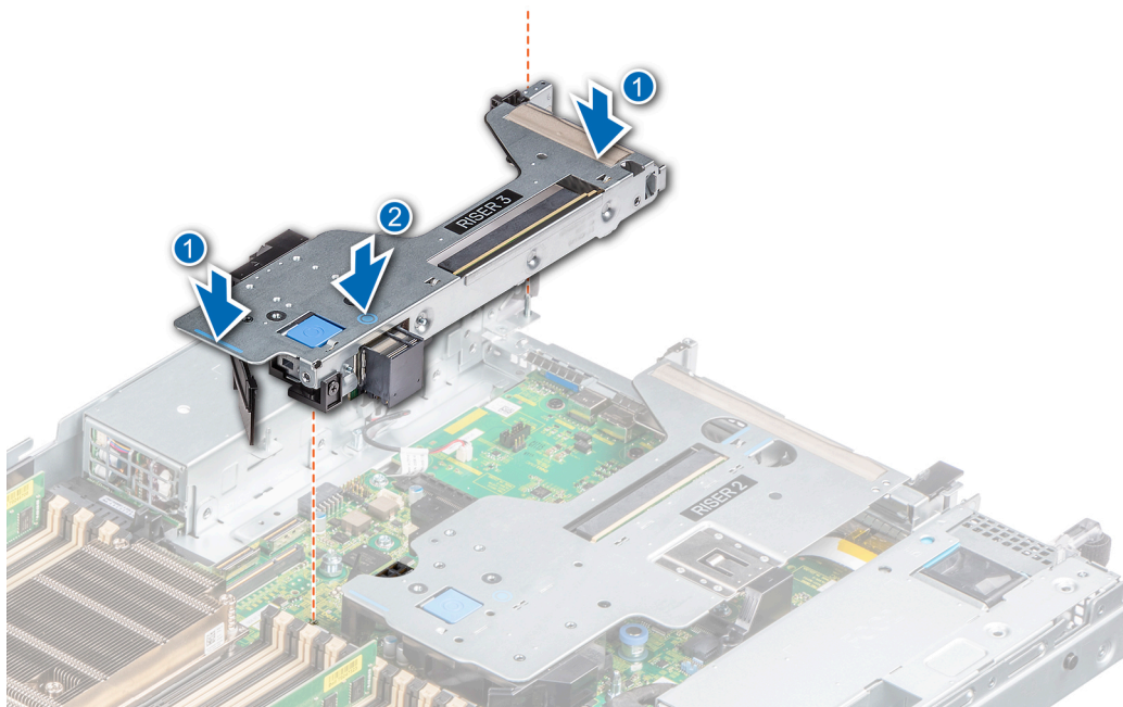
Abbildung 89. Installieren des Erweiterungskarten-Risers (Riser 3)
