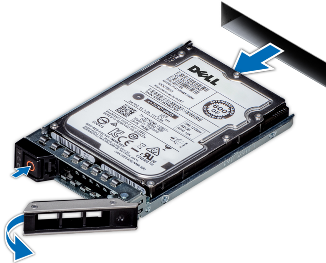
Abbildung 35. Entfernen eines Festplattenträgers
