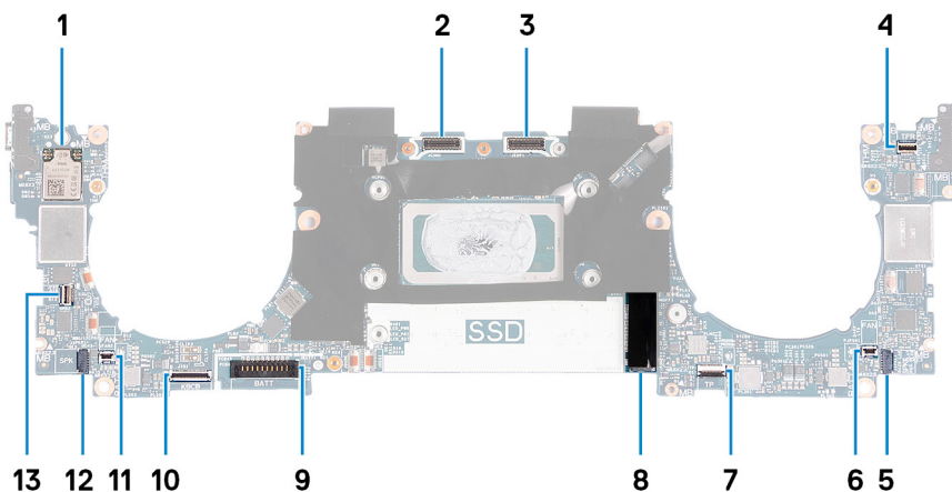
Abbildung 1. Systemplattenanschlüsse
