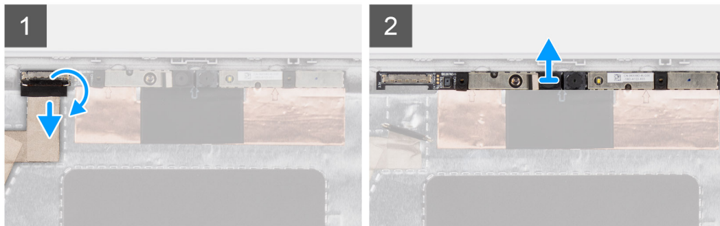
Abbildung 2. Entfernen des Infrarot-Kameramoduls
