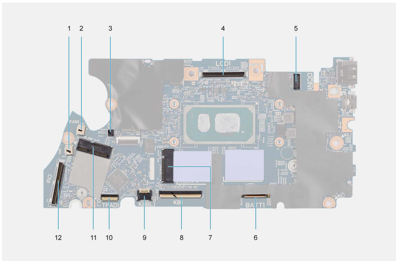
Afbeelding 2. Systeemkaartconnectoren
