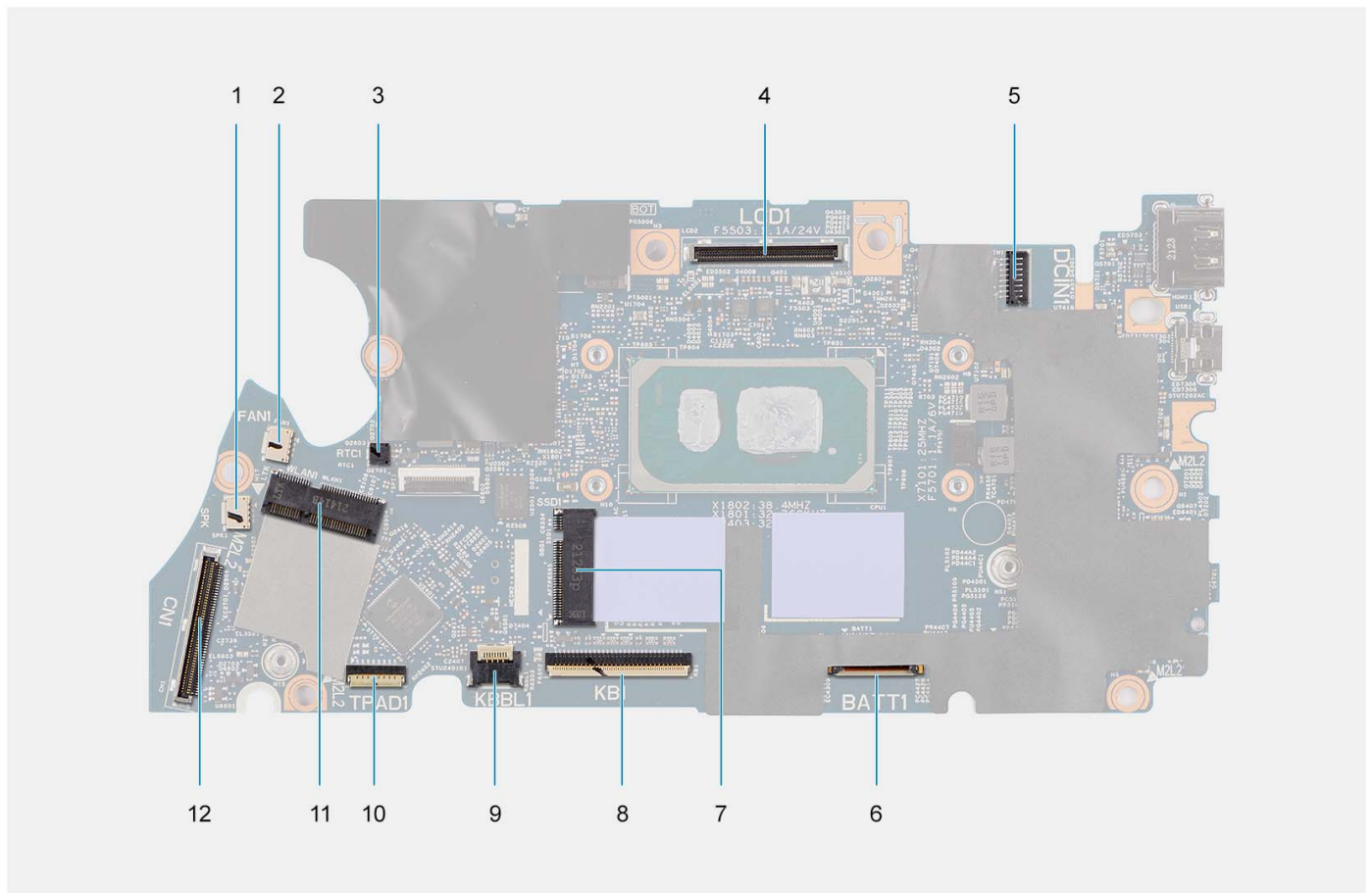
Afbeelding 1. Systeemkaartconnectoren
