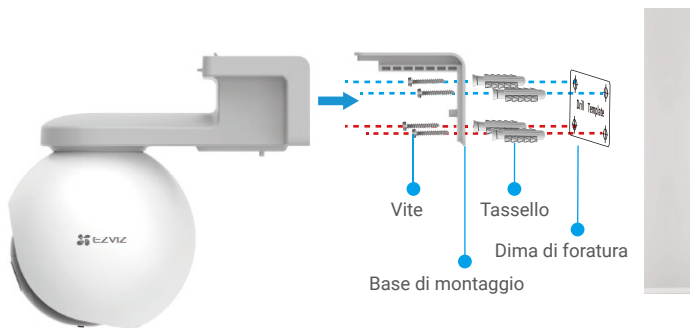
Fig. 2 Montaggio a parete
