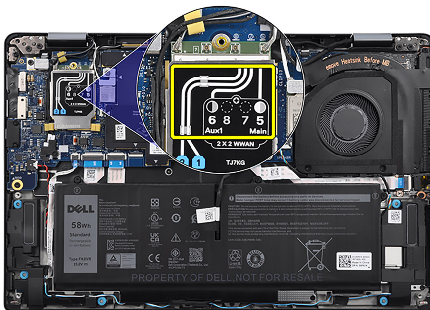
Figura 1. Configurazione WWAN 4G
